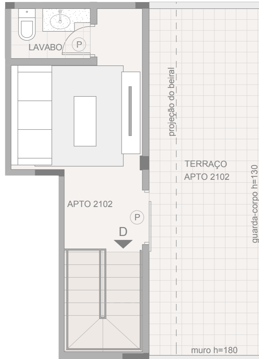
2º NÍVEL • 21º PAVIMENTO
