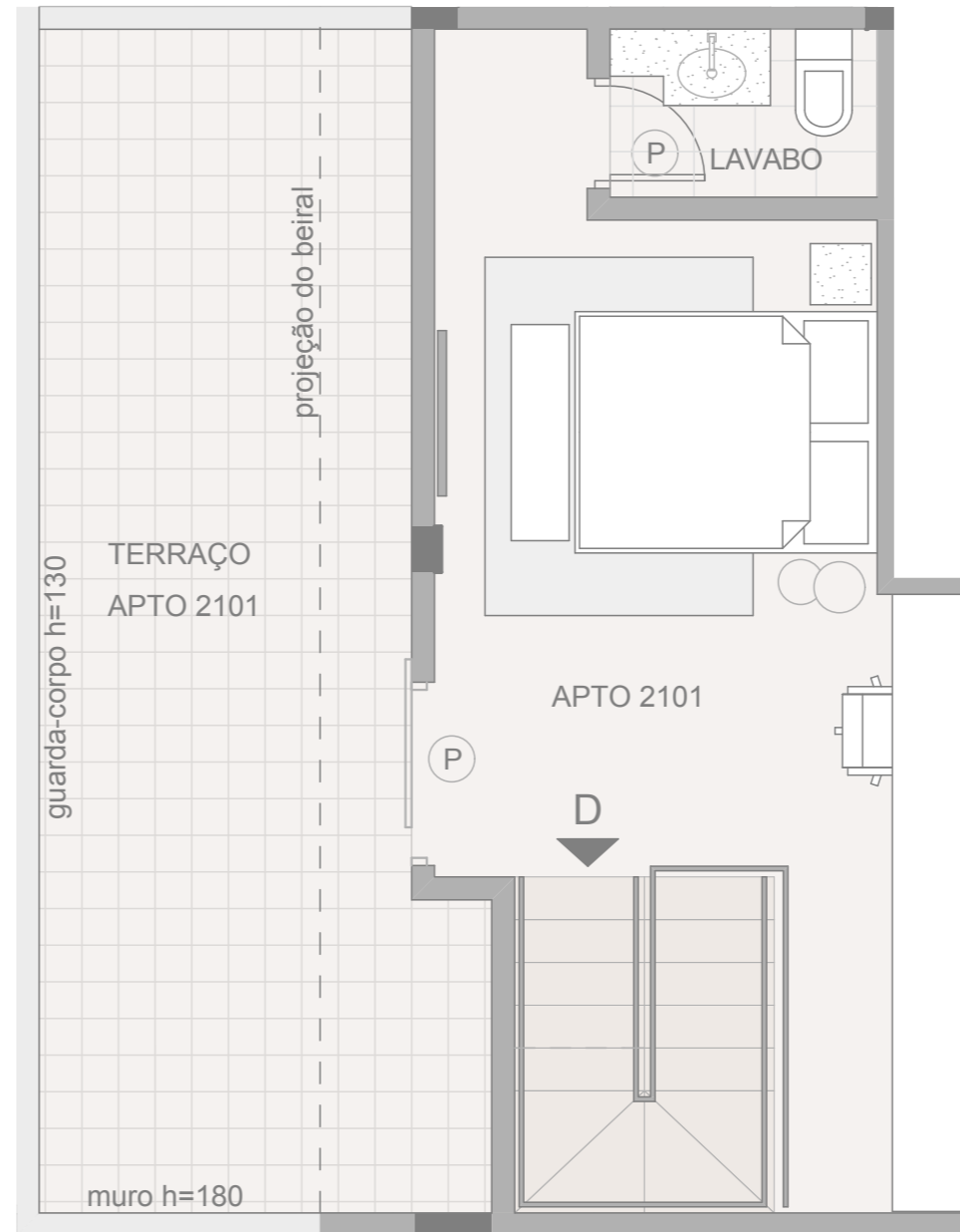
2º NÍVEL • 21º PAVIMENTO
