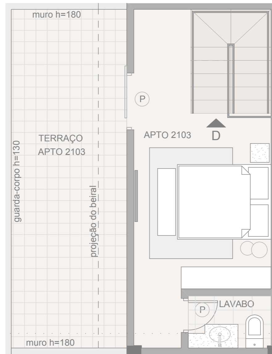
2º NÍVEL • 21º PAVIMENTO
